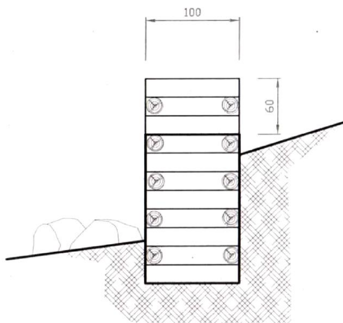
SEZIONE LATERALE
