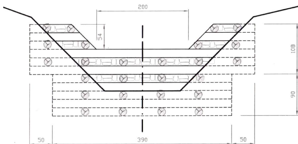
SEZIONE FRONTALE
